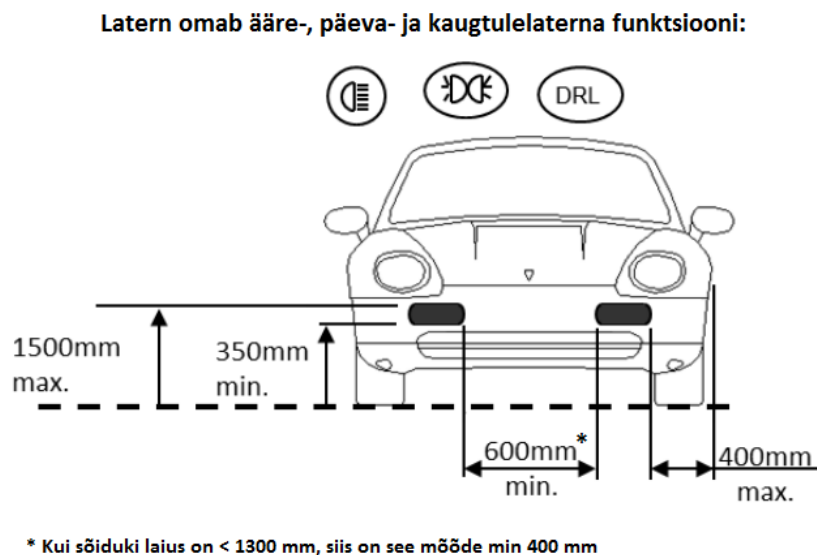
Joonis 1: Väljavõte Lazer Lamps Ltd. tulelaternate paigaldusjuhiseist
