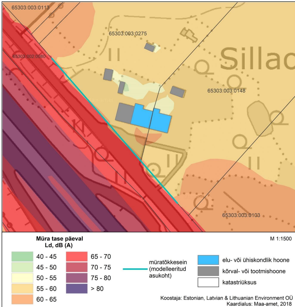
Joonis 7. Sillaotsa müra tõkkesein. Ld
