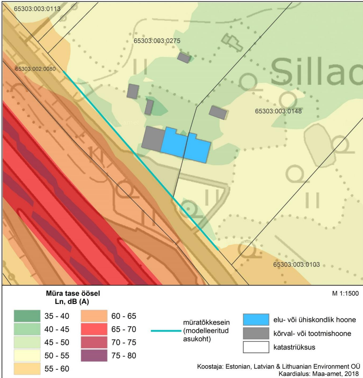
Joonis 8. Sillaotsa müratõkkesein. Ln
