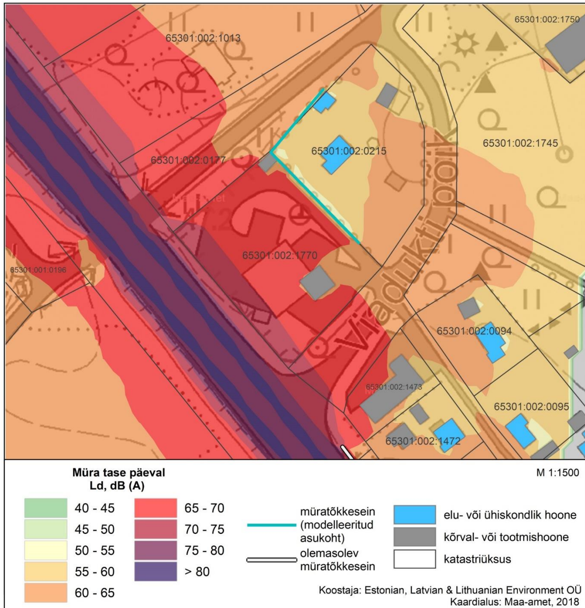
Joonis 5. Viadukti põik 2 müratõkkesein. Ld
