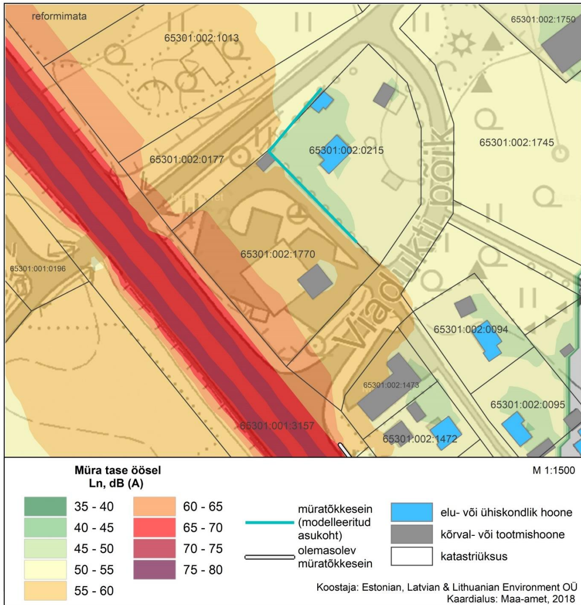
Joonis 6. Viadukti põik 2 müratõkkesein. Ln
