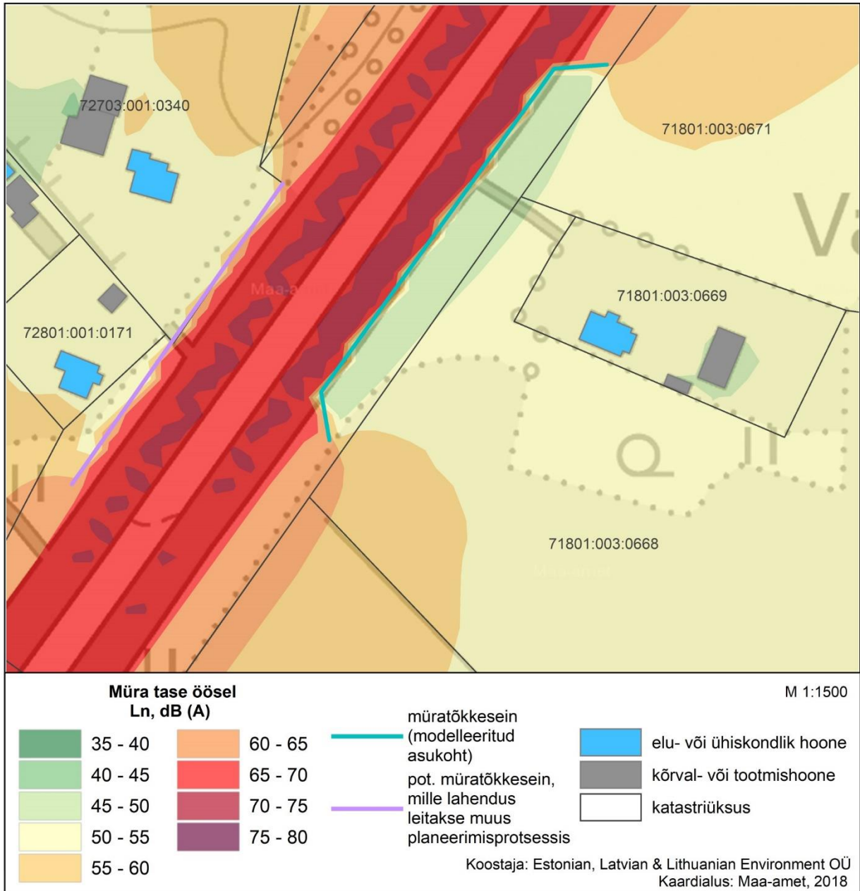
Joonis 12. Varju müratõkkesein. Ln
