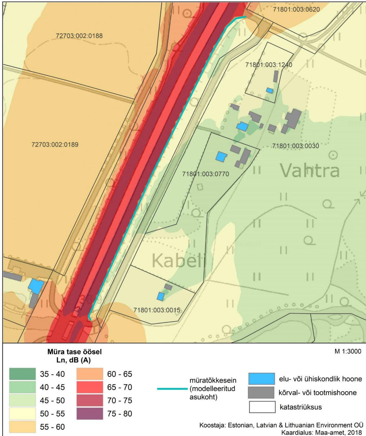
Joonis 14. Salme, Vahtra, Oja, Kabeli müratõkkesein. Ln
