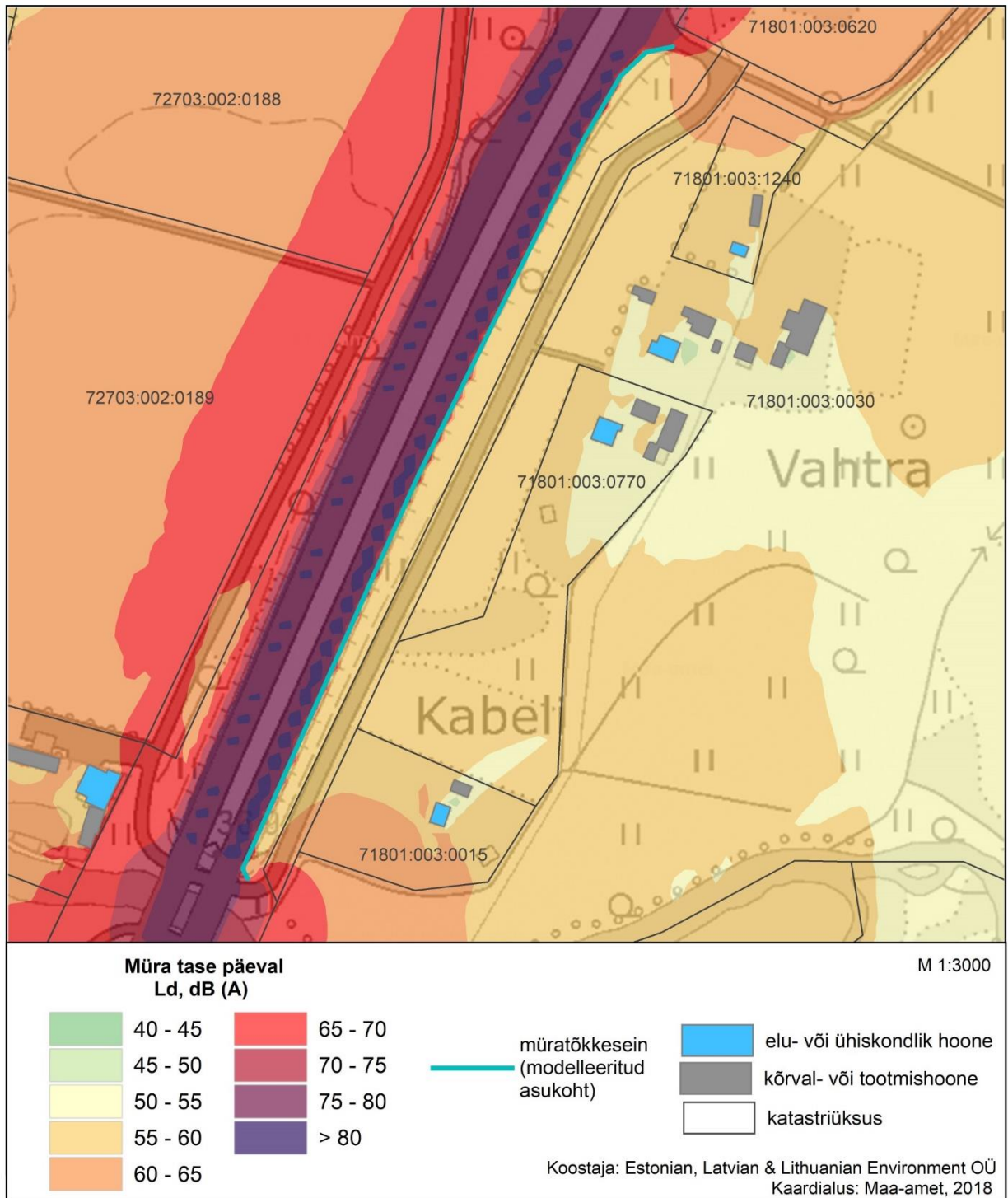
Joonis 13. Salme, Vahtra, Oja, Kabeli müratõkkesein. Ld
