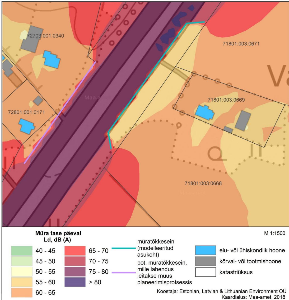
Joonis 11. Varju müratõkkesein. Ld
