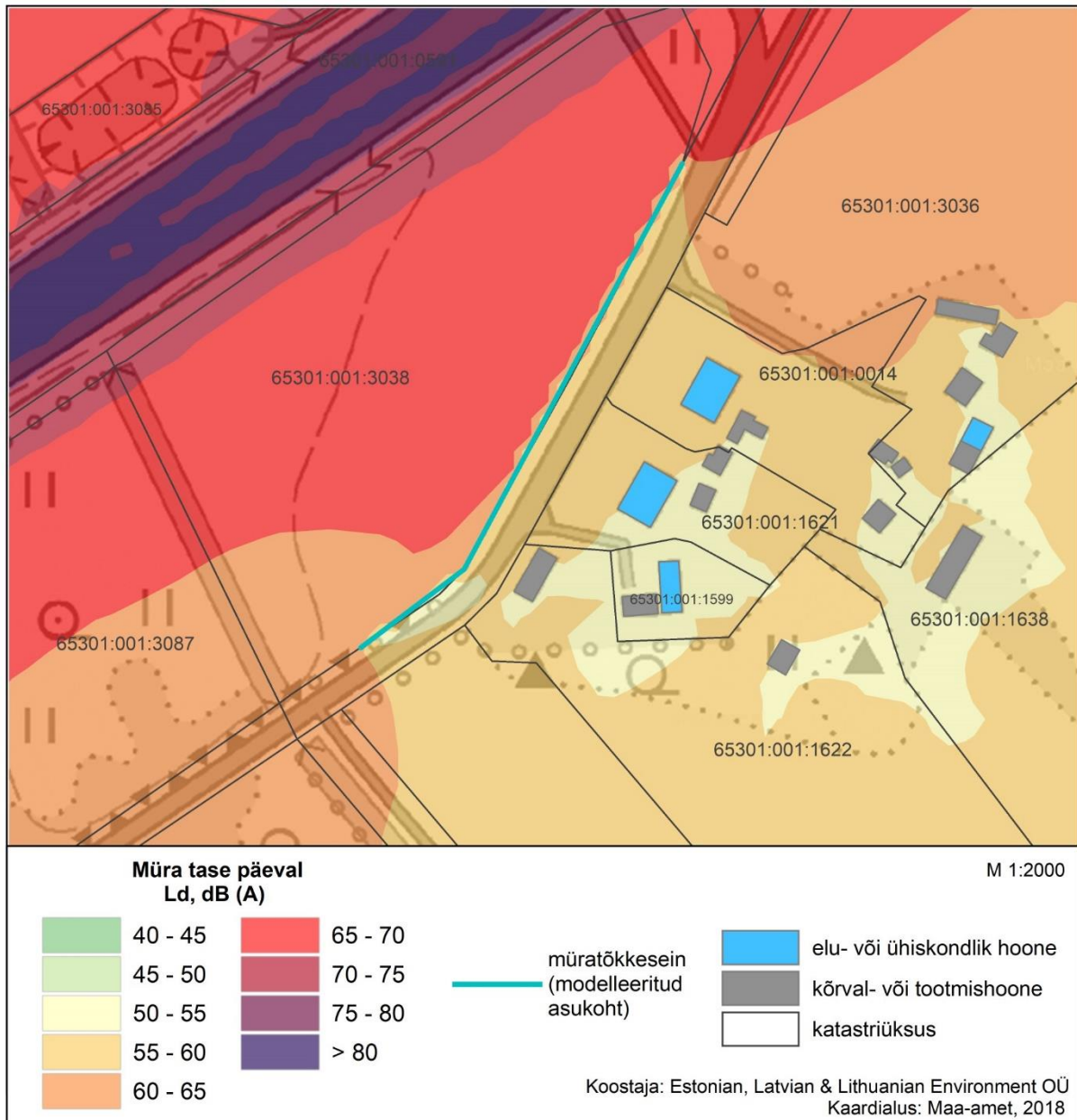
Joonis 25. Õlleköögi 1 ja 3 müratõkkesein. Ld
