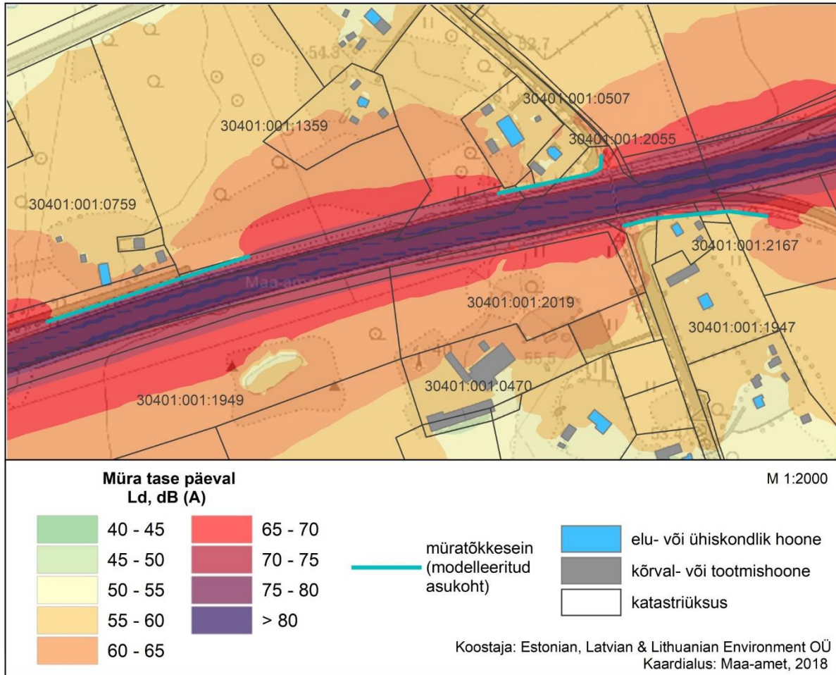
Joonis 27. Mikuhansu 17, Kangru 17 ja Vaela 44 müra tõkkesein. Ld
