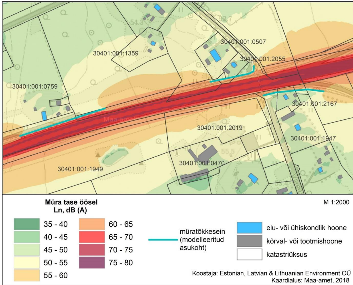
Joonis 28. Mikuhansu 17, Kangru 17 ja Vaela 44 müratõkkesein. Ln
