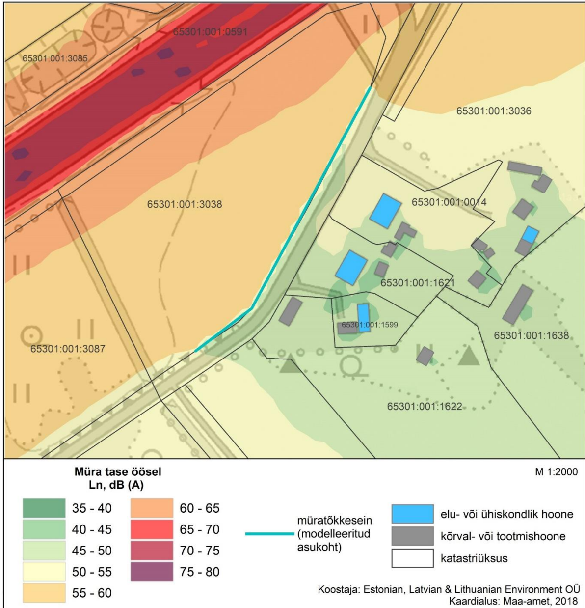
Joonis 26. Õlleköögi 1 ja 3 müratõkkesein. Ln
