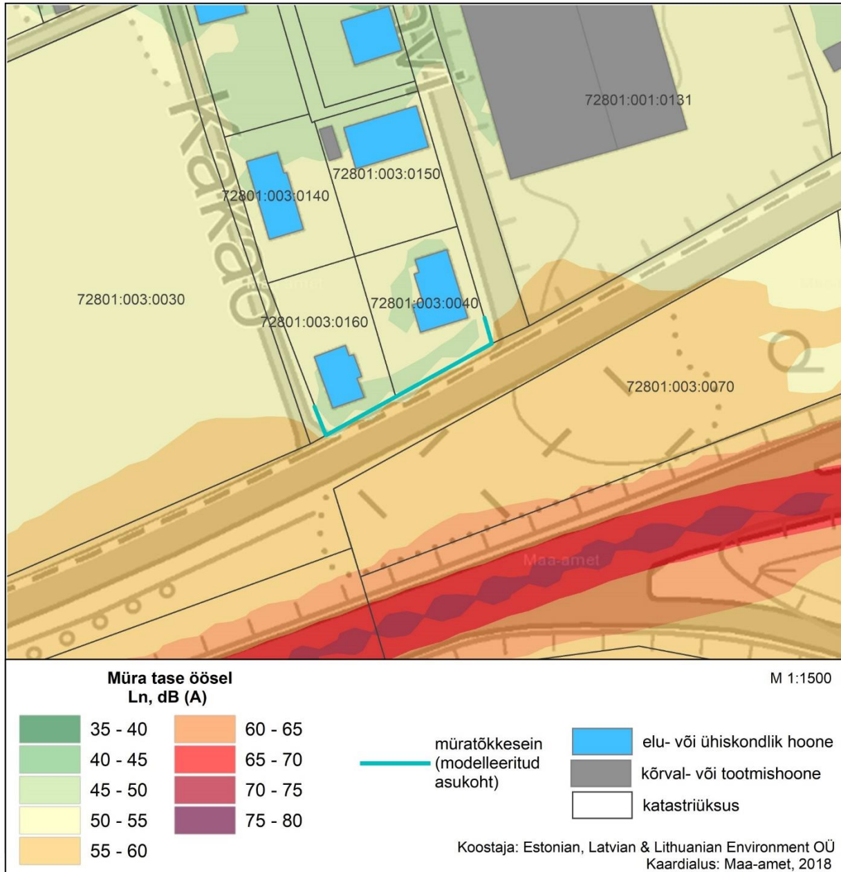
Joonis 30. Kohvi tn 2 ja Kakao tn 1 müratõkkesein. Ln
