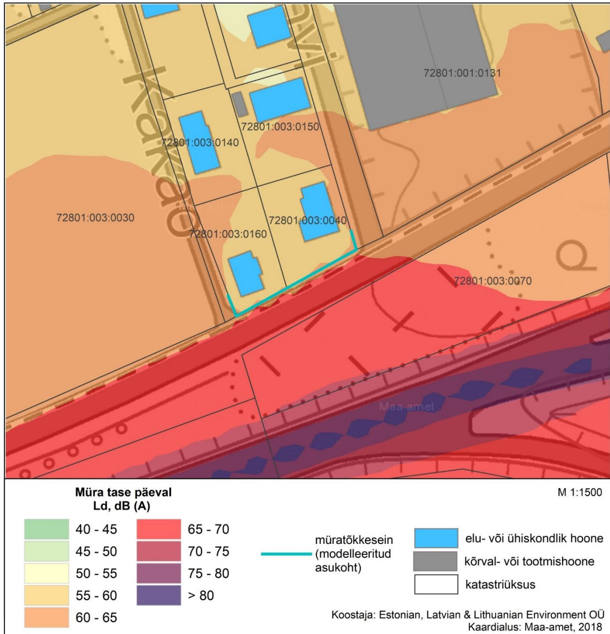
Joonis 29. Kohvi tn 2 ja Kakao tn 1 müratõkkesein. Ld
